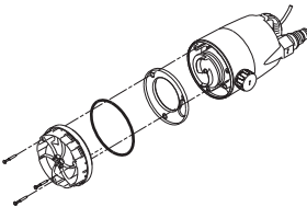
Рис. 13 Снятие нижней части
